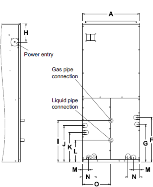
Left side
